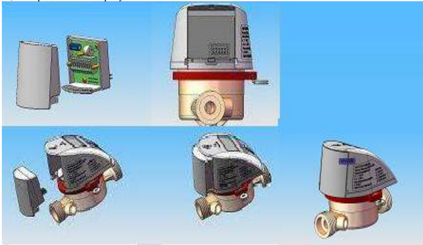
Рисунок 2. Размещение интерфейса
