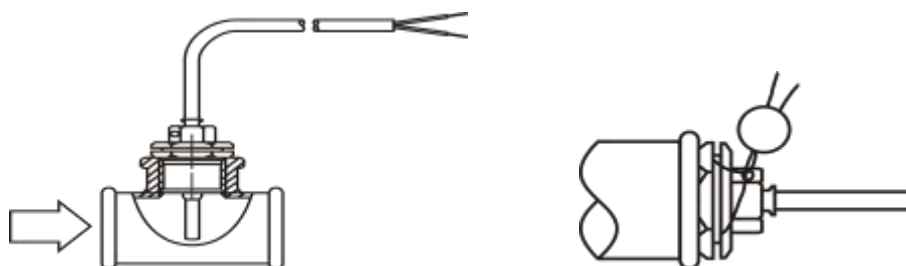
Рис.4 Монтаж и пломбирование термopеобразователя сопротивления в штуцере при помощи ниппеля.
