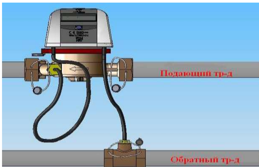
Рис.3 Монтаж теплосчетчика (монтаж термopеобразователя сопротивления в тройнике)
